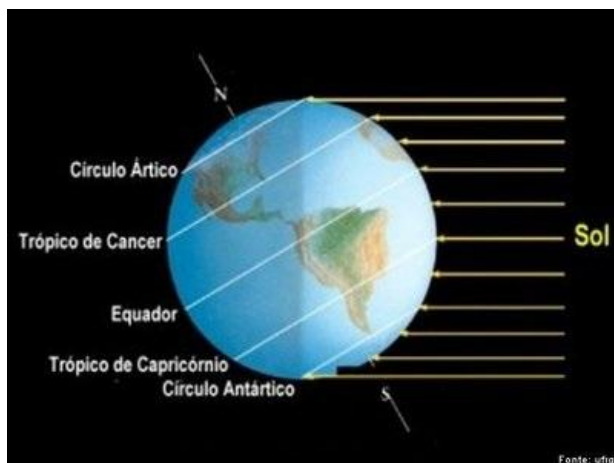
Fig. 4 - Raios de luz oriundos do Sol chegam a Terra praticamente paralelos. Podemos observar que o eixo de rotação é inclinado em relação à órbita de translação.
