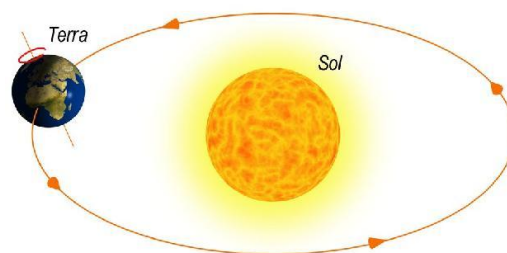
Fig. 1 - A Terra tem uma órbita elíptica com uma excentricidade bem pequena.
