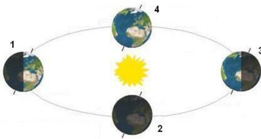
Fig. 6 – Representação do sistema Terra-Sol, com detalhes para o eixo de rotação da Terra que sempre aponta na mesma direção.
